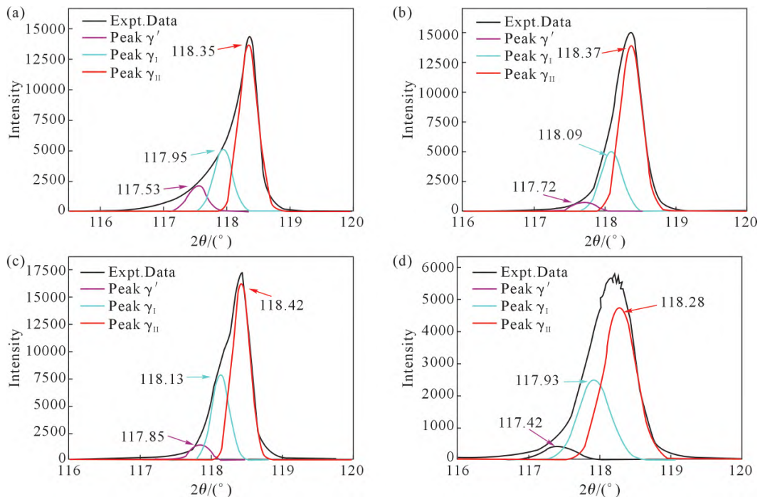
图 6 DD10 单晶合金 1 100 °C 热暴露不同时间后测定的 XRD 扫描图:(a) 热处理态;(b) 200 h;(c) 300 h;(d) 500 h Fig.6 XRD scans of the single-crystal superalloy after thermal exposure at 1 100 °C: (a) heat-treated; (b) 200 h; (c) 300 h; (d) 500 h
