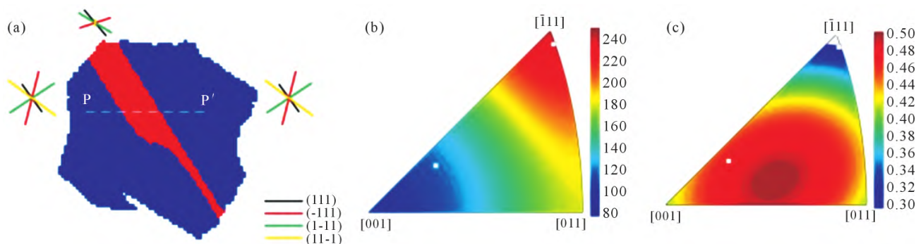
图9 用于孪晶界分析的晶粒:(a)含有退火孪晶的晶粒形貌。孪晶与母晶对的对应 \{111\} 滑移迹线以不同颜色绘制,线的长度表示施密特因子的相对大小;(b) \{111\}<110> 滑移系沿载荷方向的弹性模量;(c) \{111\}<110> 滑移系沿载荷方向的施密特因子 [64]
