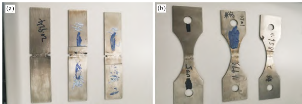
图 6 室温及高温低周疲劳试样:(a) 室温( K_f=3 );(b) 高温( K_f=1 )
