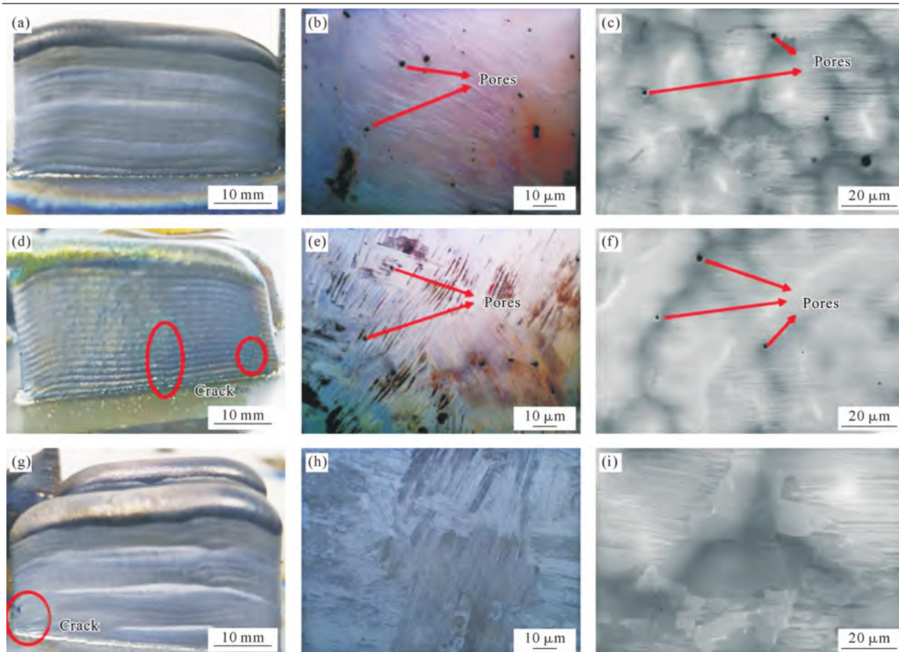
图4 高Nb-TiAl合金薄壁件及金相组织:(a~c)工艺3;(d~f)工艺4;(g~i)工艺5
