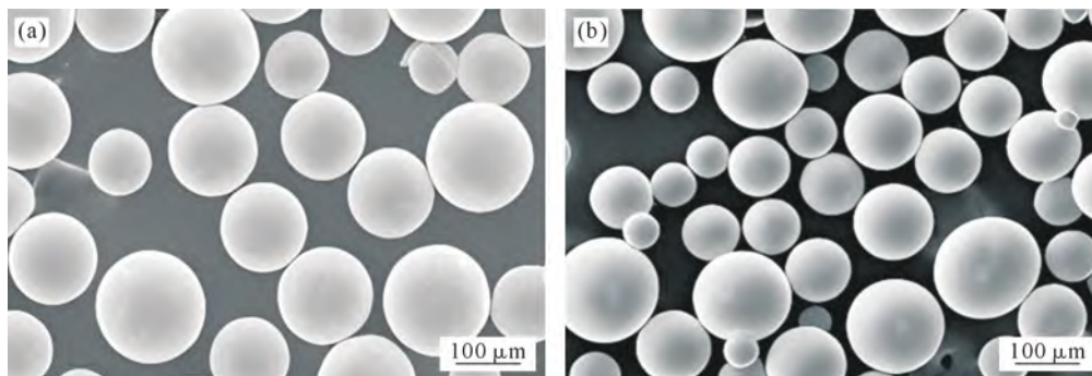
图1 原始合金粉末的SEM图像:(a) Ti60; (b) Ti-45Al-8Nb
