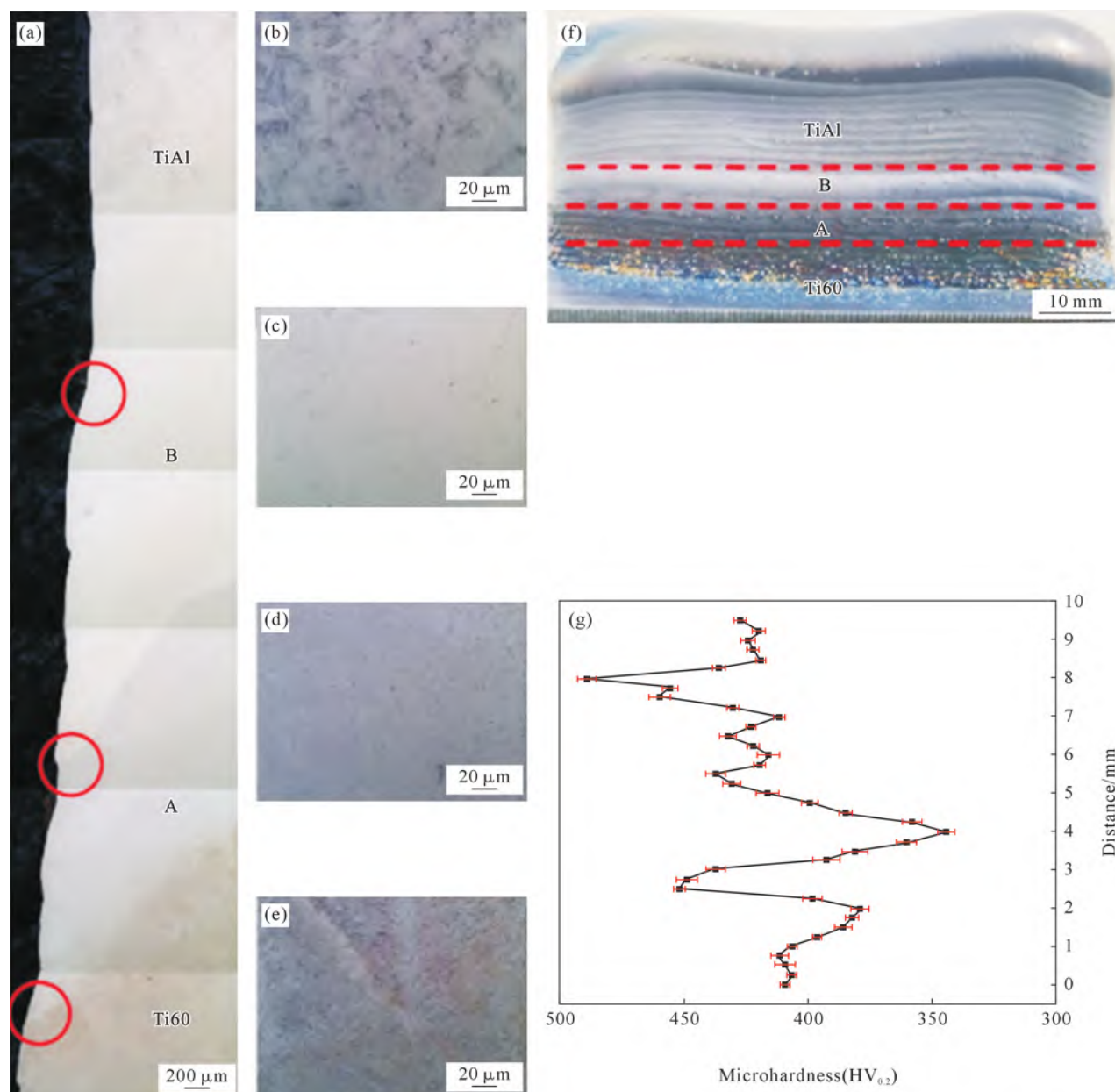
图 10 梯度过渡沉积 Ti/A/B/TiAl 合金功能梯度材料:(a) 界面形貌;(b) TiAl 合金组织;(c) 过渡区 A 中心组织;(d) 过渡区 B 中心组织;(e) Ti60 合金组织;(f) FGM 宏观形貌;(g) 界面显微硬度
