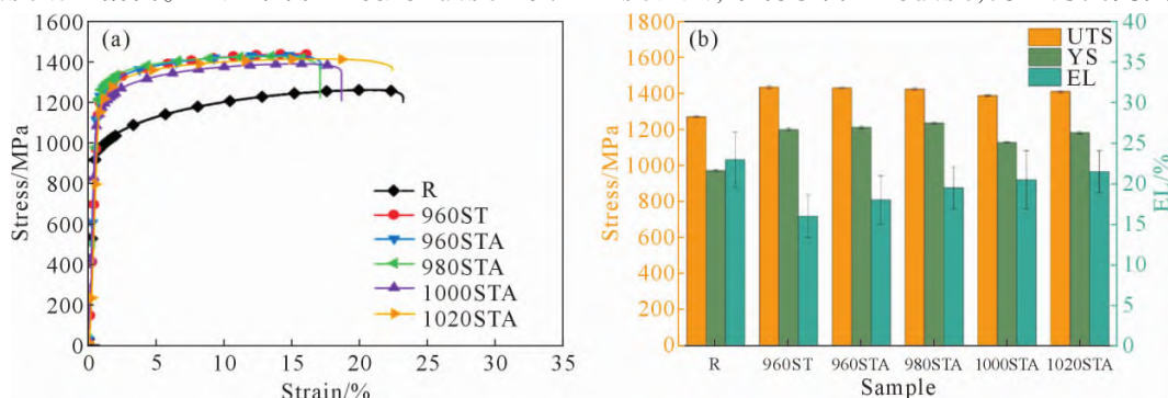
图5 室温下不同热处理态合金拉伸性能:(a) 应力-应变曲线;(b) 抗拉强度、屈服强度及伸长率
