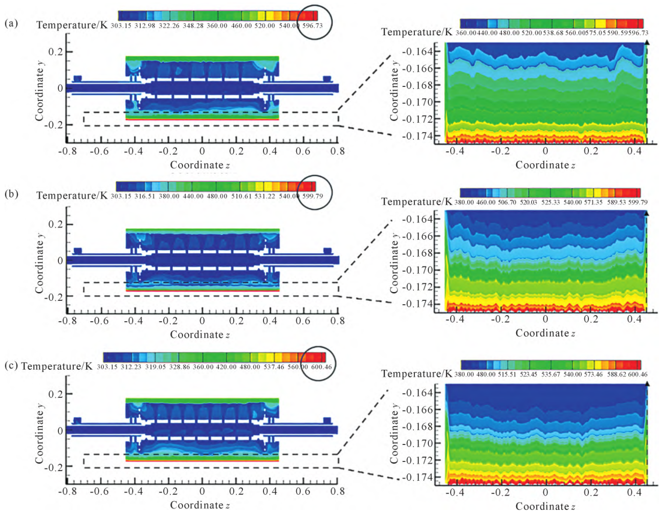
图5 x=0 处截面水冷辊温度分布云图:(a) 24个;(b) 28个;(c) 32个
