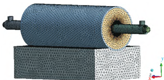
图4 连铸区有限元网格划分结果
