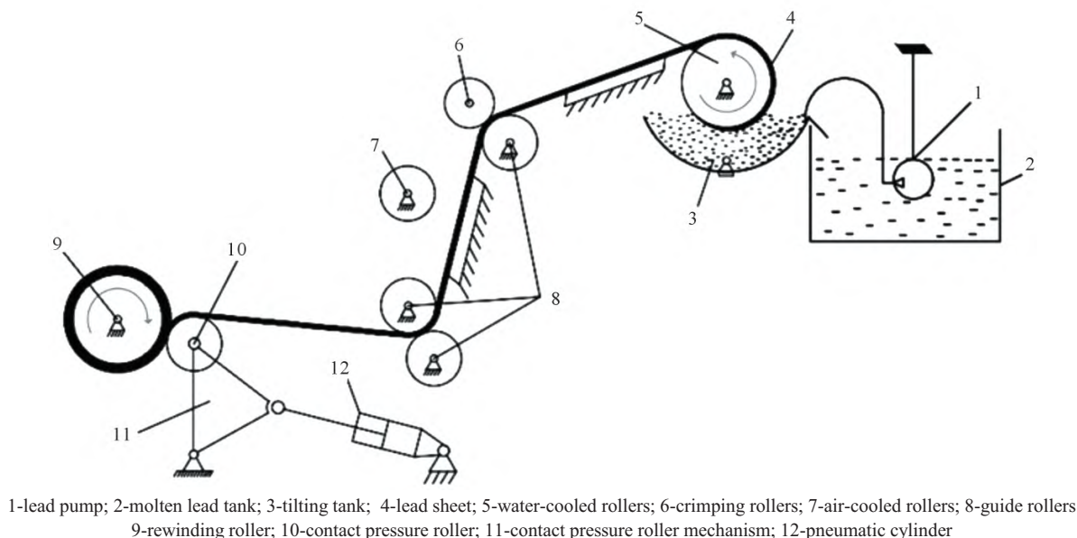
图 1 铅薄板单辊连铸机工作原理
