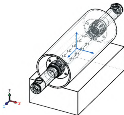
图3 连铸区几何模型
