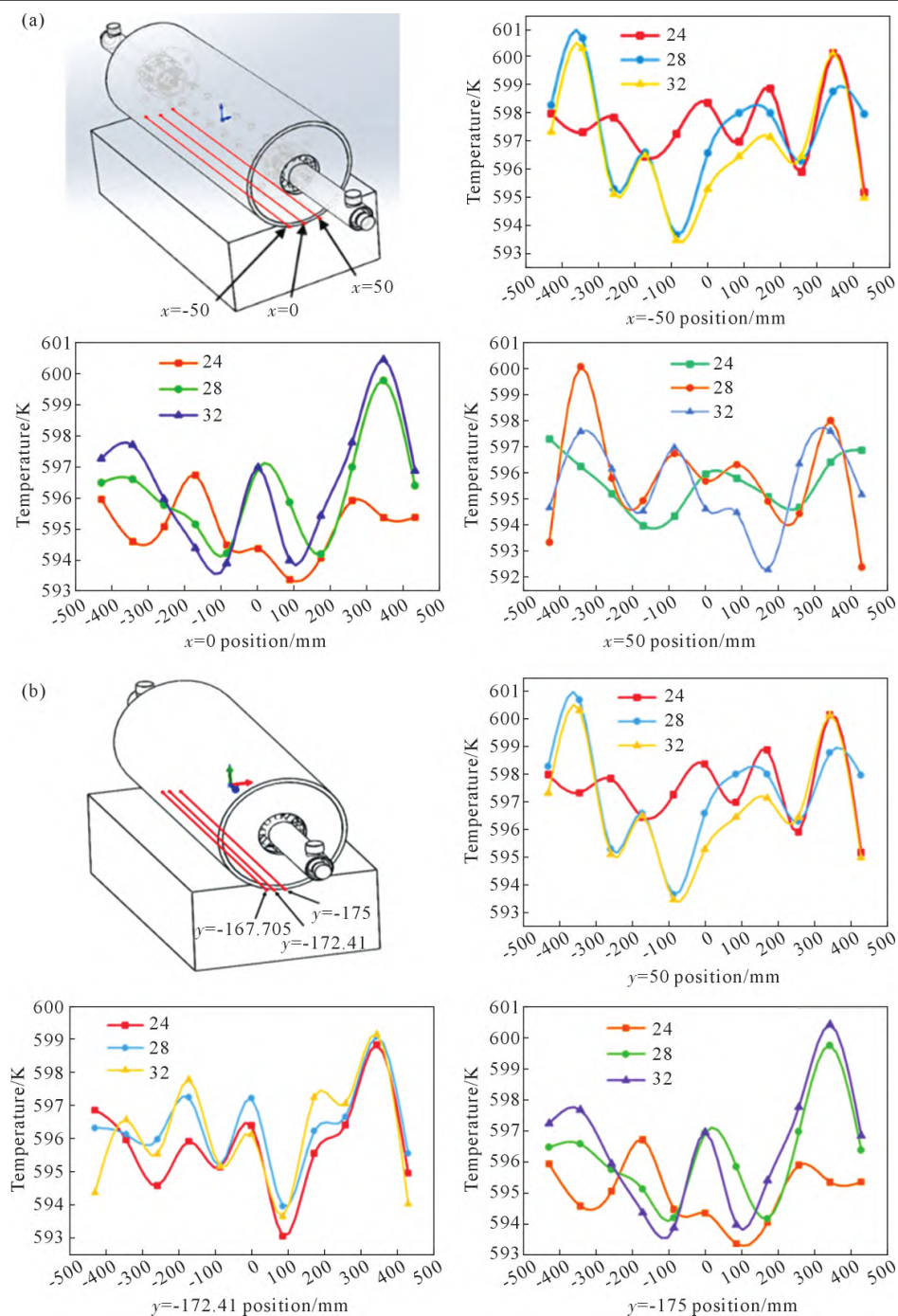
图 8 不同位置铅辊接触壁面同一水平线温度分布:(a) 不同横坐标;(b) 不同纵坐标
