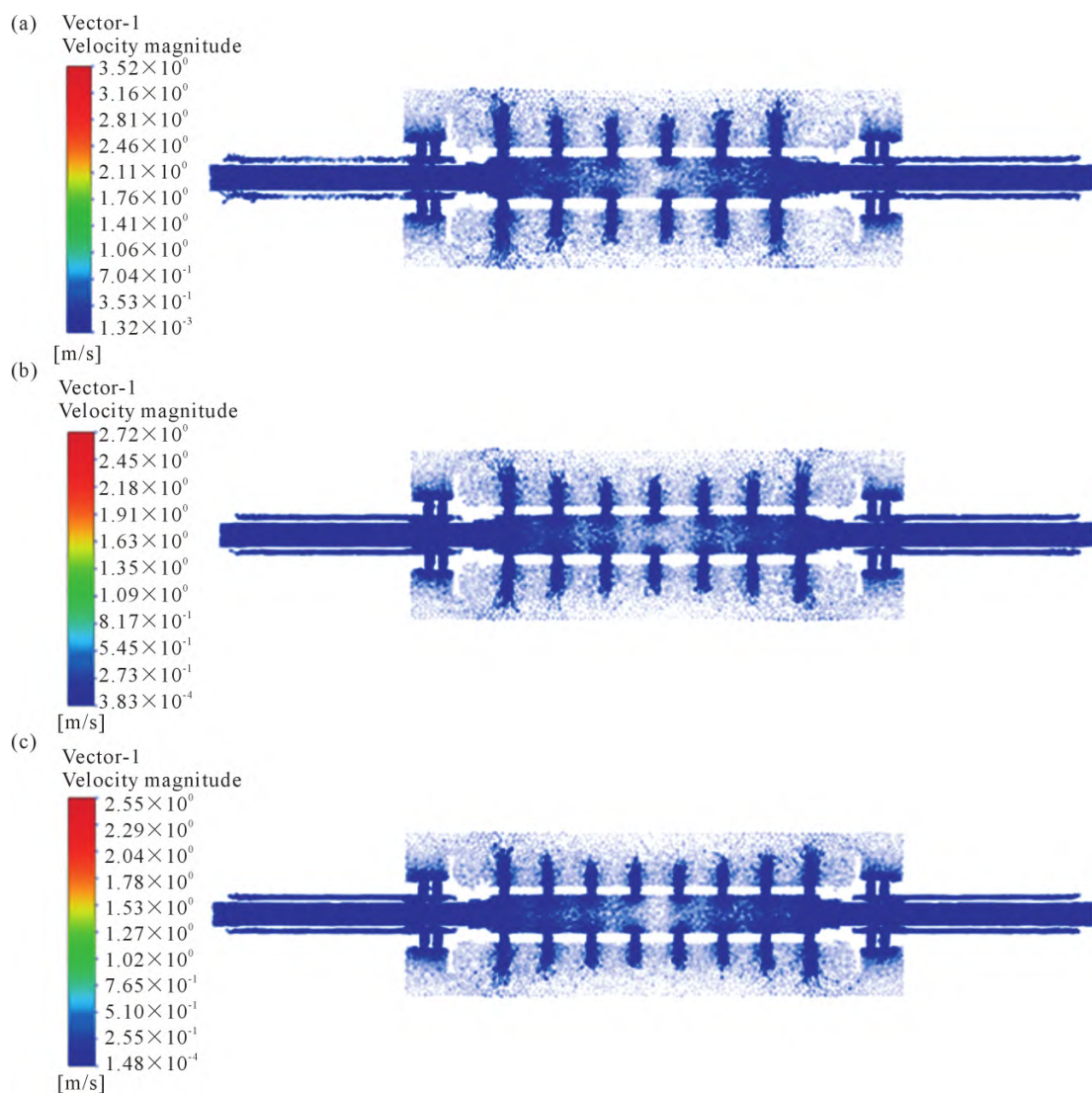
图7 y=0 处截面不同水孔数目对应速度矢量分布:(a) 24个;(b) 28个;(c) 32个
