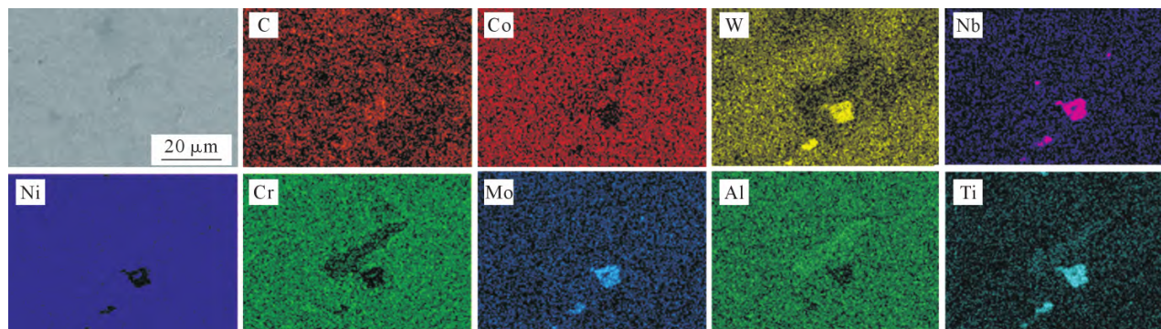
图7 铸态 K465 合金中碳化物 EDS 分析 Fig.7 EDS analysis of carbides in the as-cast K465 alloy
