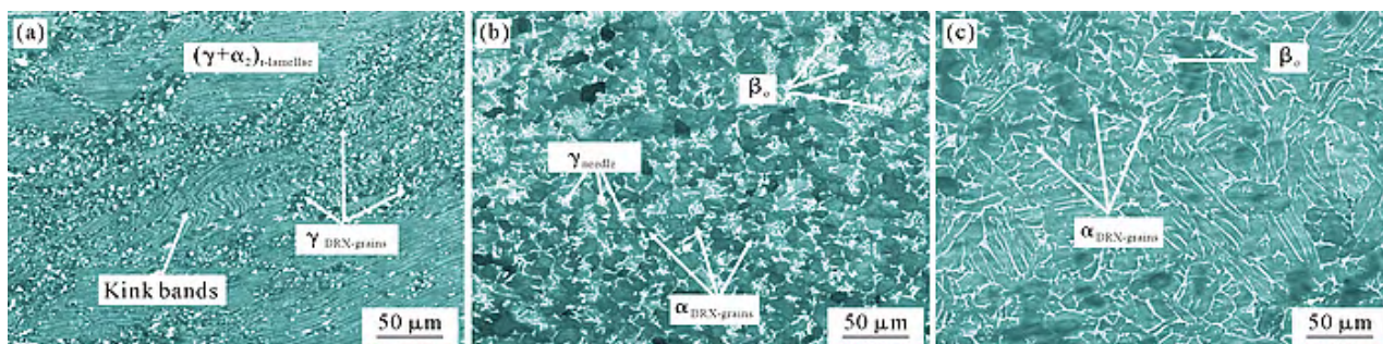
图3 TRC-1.5合金在不同温度下热压缩后的微观组织图:(a) 1 150 ^{\circ}\text{C} ; (b) 1 200 ^{\circ}\text{C} ; (c) 1 250 ^{\circ}\text{C}
