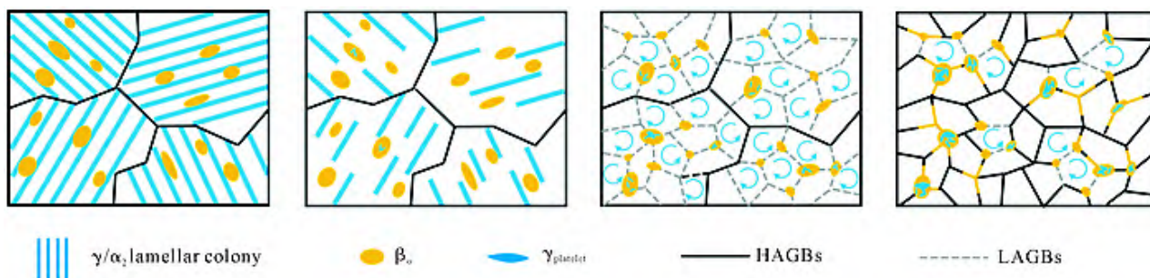
图9 TRC-1.5合金在1200 °C/0.01 s -1 热变形条件下的微观组织演变示意图 Fig.9 Microstructure evolution of the TRC-1.5 alloy deformed at 1200 °C/0.01 s -1
