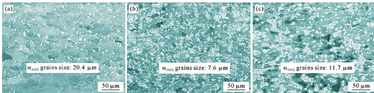
图 4 TRC- x(x=1, 1.5, 2) 合金在 1 200 °C/0.01 s -1 /60%条件下热变形的微观组织:(a) 1%; (b) 1.5%; (c) 2%
