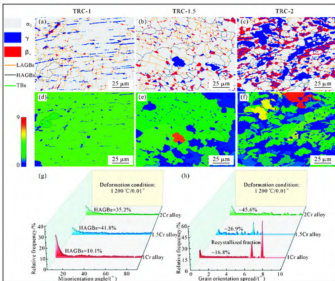
图 5 TRC- x(x=1, 1.5, 2) 合金在 1 200 °C/0.01 s -1 热变形条件下应变量为 40%微观组织 EBSD 分析:(a~c) 相与晶界图;(d~f) GOS 图;(g) 晶界分布;(h) GOS 分布
