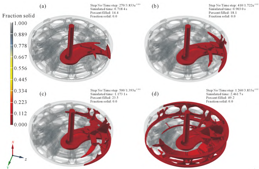
图 3 单股进水方案模拟结果:(a) 金属液进入铸件型腔;(b) 金属液在支板处汇流;(c) 金属液沿横浇道充型;(d) 金属液在另一处汇流
