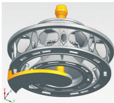
图 2 单股进水方案
