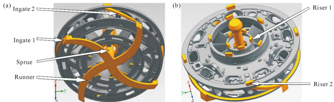
图4 4股进水工艺方案
