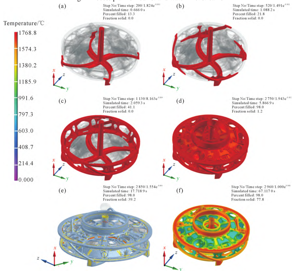
图5 4股进水模拟结果:(a)金属液沿横浇道到达外沿阶段;(b)金属液从内浇口进入铸件阶段;(c)金属液进行向心充型阶段;(d)金属液完全充满;(e)固相率;(f)热节区域
