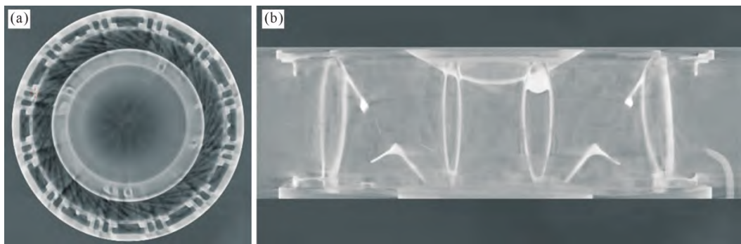
图 6 铸件工业 CT:(a) 俯视图;(b) 主视图
