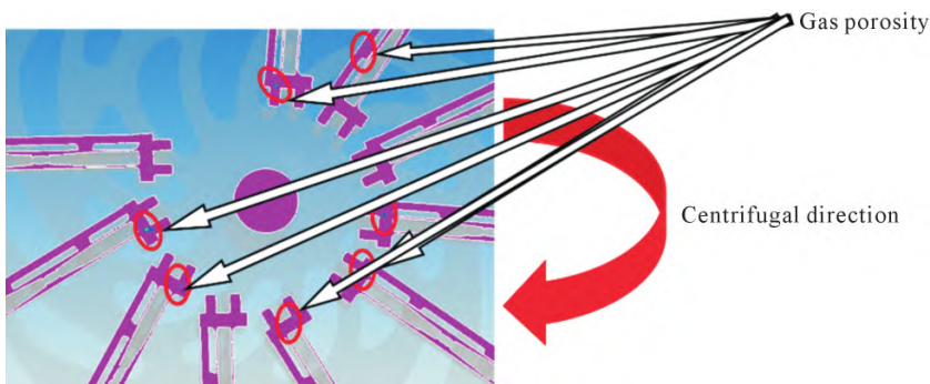
图 4 缺陷模拟结果 Fig.4 Simulation results of defects
