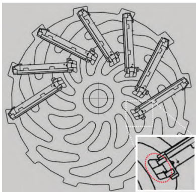
图 5 工艺优化示意图 Fig.5 Schematic diagram of process optimization
