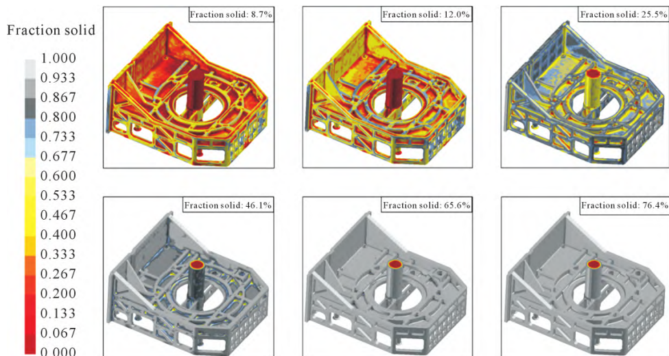
图5 安装支架凝固过程
