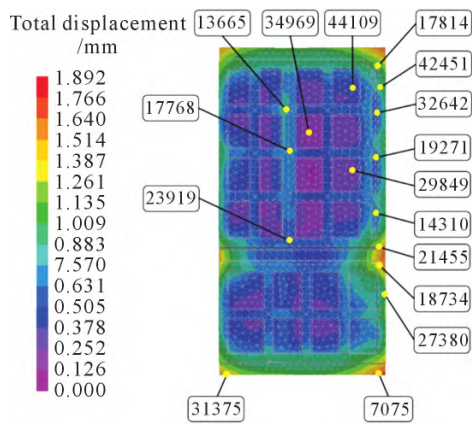
图 10 安装支架标定面所选特征点
