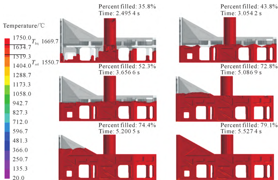
图 4 安装支架充型过程
