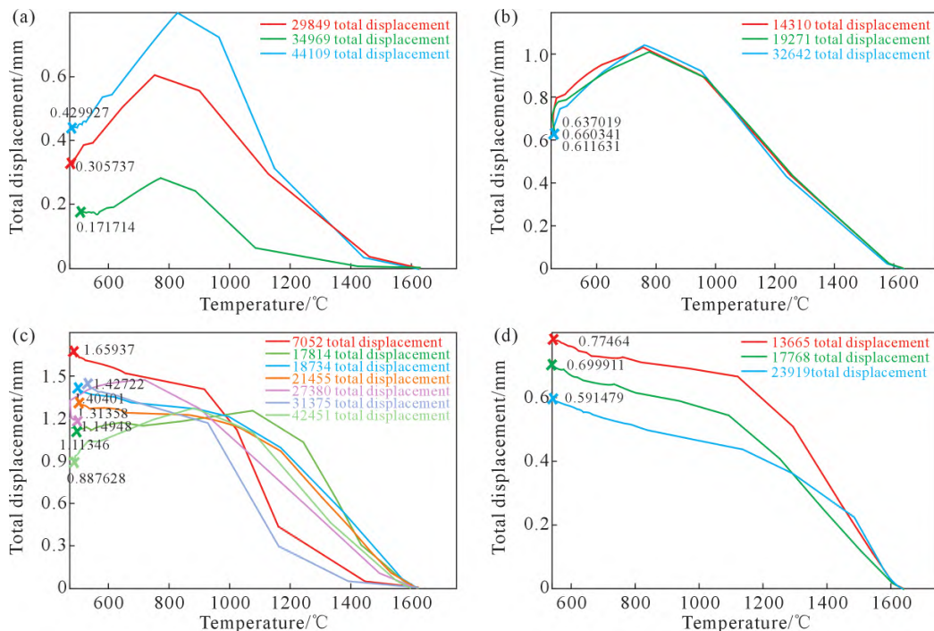
图 11 安装支架标定面所选特征点变形量:(a) E-E 平面;(b) F-F 平面;(c) G-G 平面;(d) H-H 平面
