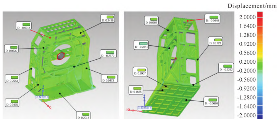
图 12 安装支架预变形控制结果
