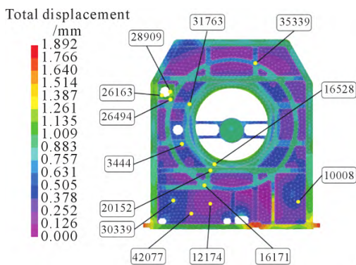
图 8 安装支架标定面所选特征点
