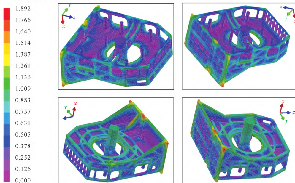
图6 安装支架变形结果
