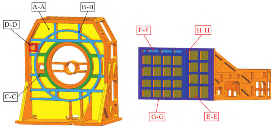
图 7 安装支架标定面
