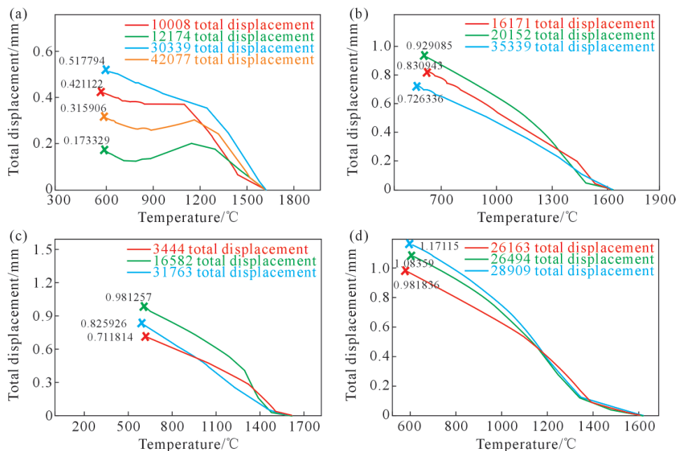
图 9 安装支架标定面所选特征点变形量: (a) A-A 平面; (b) B-B 平面; (c) C-C 平面; (d) D-D 平面
