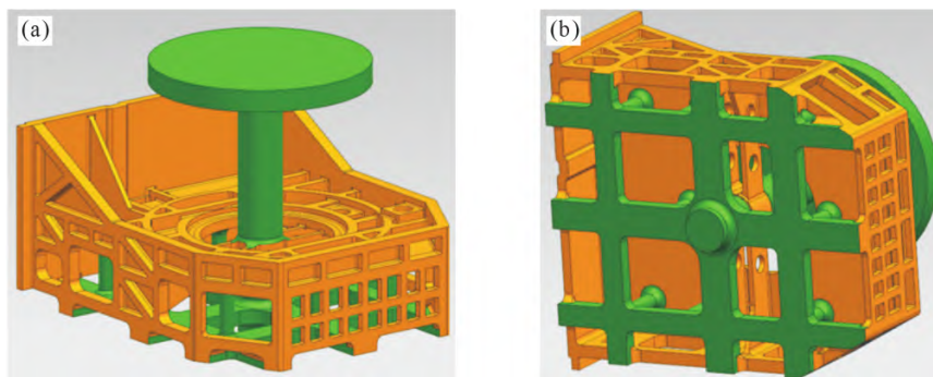
图 2 安装支架浇注系统:(a) 主视图;(b) 侧视图
