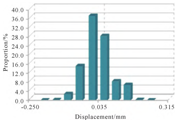
图 13 安装支架变形量偏差分布
