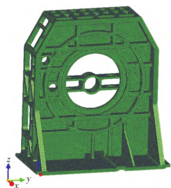
图 3 安装支架网格划分
