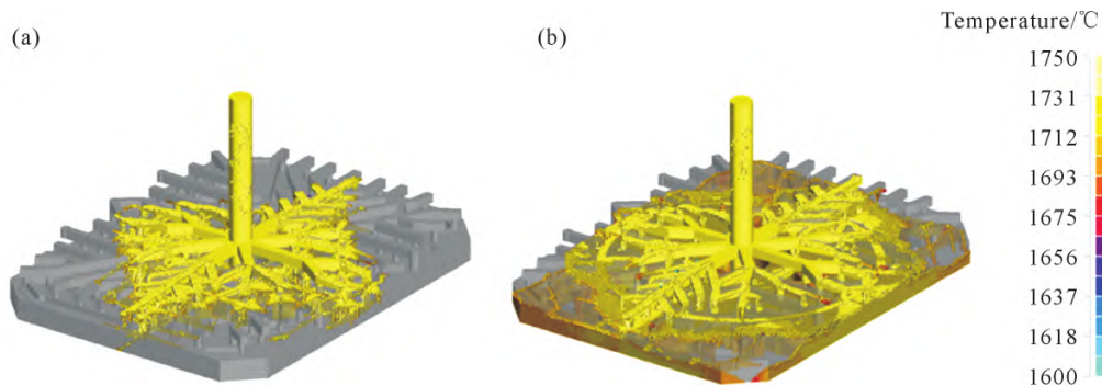
图6 雨淋式浇注系统充型过程温度场变化:(a) 2 s; (b) 5 s
