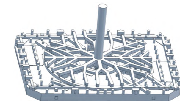
图8 优化后的雨淋式浇注系统
