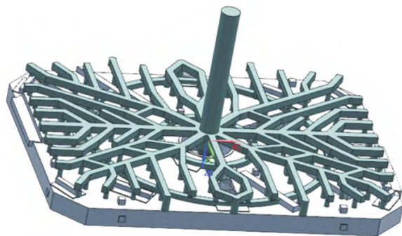
图 5 雨淋式浇注系统
