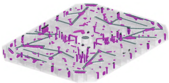
图 4 顶注式浇注系统缩松缩孔缺陷模拟预测
