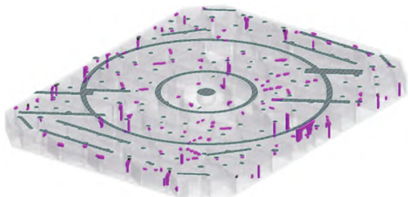
图7 雨淋式浇注系统缩孔缩松缺陷模拟预测
