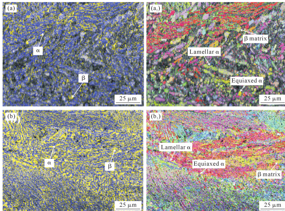
图5 变形量为60%,应变速率为 0.001\text{ s}^{-1} 的Ti-62222钛合金不同变形温度下显微组织的相图及IPF图:(a, a 1 ) 860 °C; (b, b 1 ) 890 °C
