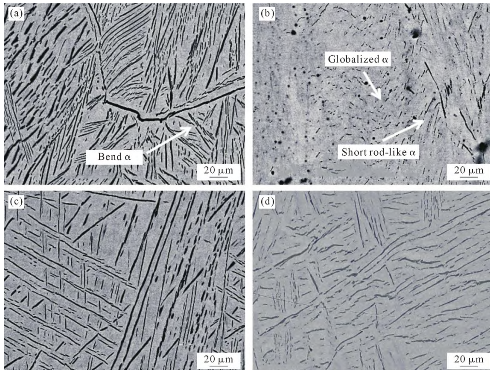
图 6 Ti-62222 钛合金在温度为 930 °C 时变形后的微观组织 : (a) 0.1 s -1 -30%; (b) 0.1 s -1 -60%; (c) 0.01 s -1 -30%; (d) 0.01 s -1 -60% Fig.6 Microstructure of Ti-62222 deformed at 930 °C: (a) 0.1 s -1 -30%; (b) 0.1 s -1 -60%; (c) 0.01 s -1 -30%; (d) 0.01 s -1 -60%
