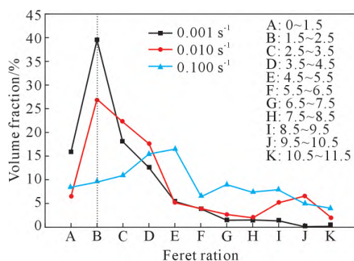
图 9 变形温度 930 °C,变形量 30%下 Ti-62222 钛合金中 \alpha 相的球化率分布
