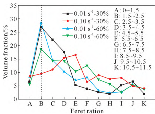
图 7 不同变形量下 Ti-62222 钛合金中 \alpha 相的球化率分布 Fig.7 Distribution of the globularization rates of Ti-62222 with different deformations
