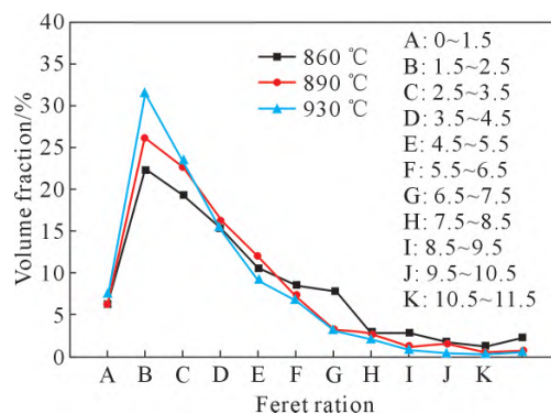
图4 不同变形温度下变形量为 60%、应变速率为 0.001 \text{ s}^{-1} 的 Ti-62222 钛合金 α 相球化率分布
