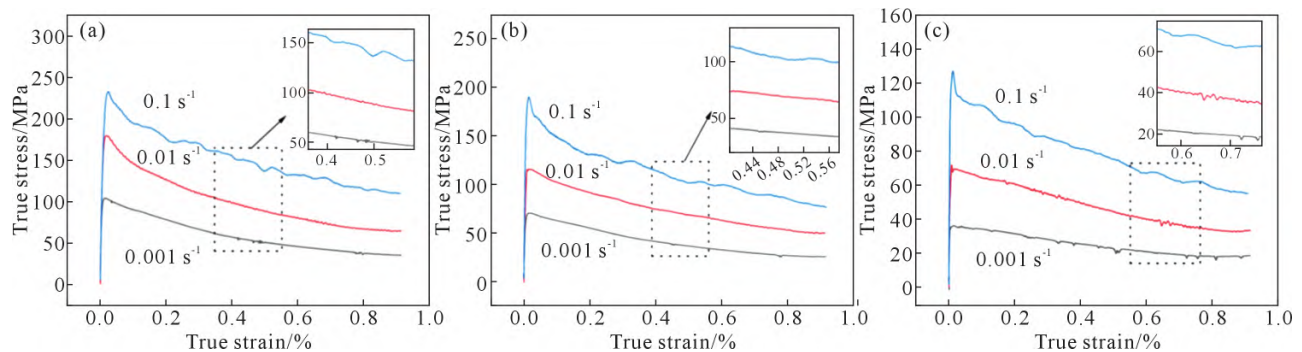
图2 Ti-62222 钛合金在不同温度下的真应力-真应变曲线:(a) 860 °C; (b) 890 °C; (c) 930 °C
