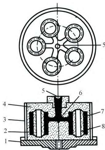
1- 旋转台; 2- 下型; 3- 砂箱; 4- 上型; 5- 中心浇道; 6- 补缩道 7- 铸件; 8- 砂芯
