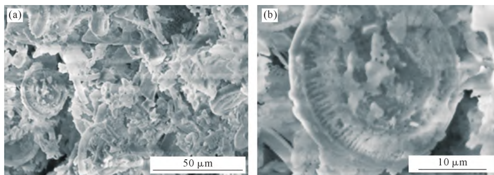
图9 硅藻土显微结构:(a) 国产;(b) 国外 [32]
