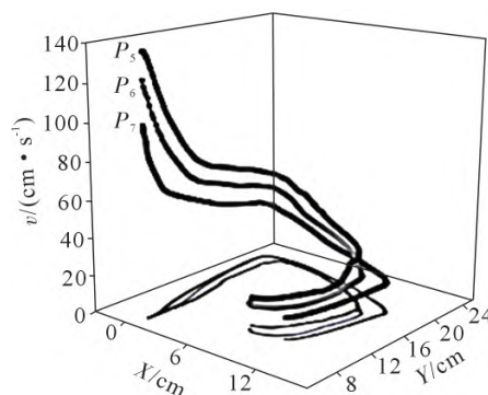
图14 不同离心转速下粒子位移-速度 [52]
