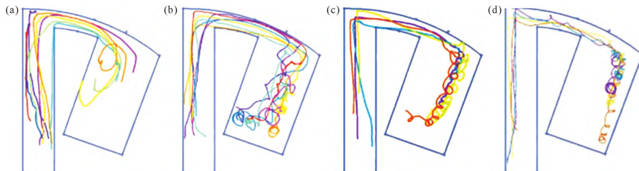
图15 不同转速下夹杂物示踪粒子运动轨迹:(a) 0 r/min; (b) 30 r/min; (c) 45 r/min; (d) 60 r/min [55]
