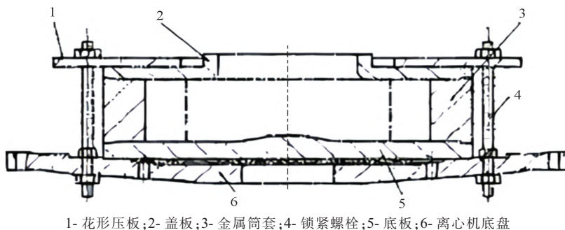
图8 立式离心机铸型、压板及锁紧装置的装配示意图 [29]
