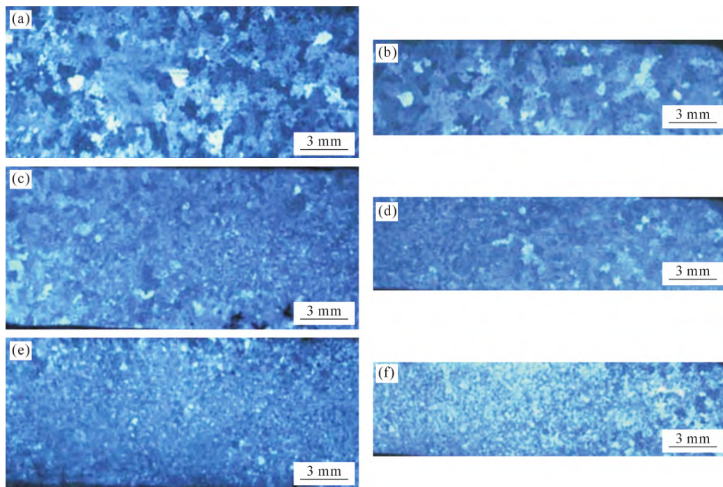
图6 不同离心转速下楔形件宏观晶粒对比:(a, b) 0 r/min; (c, d) 200 r/min; (e, f) 300 r/min [16]
