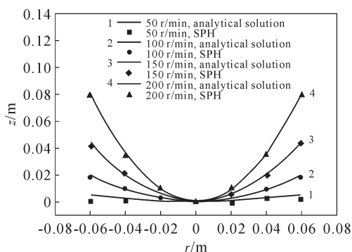
图13 自由表面解析解与SPH数值解对比 [49]
