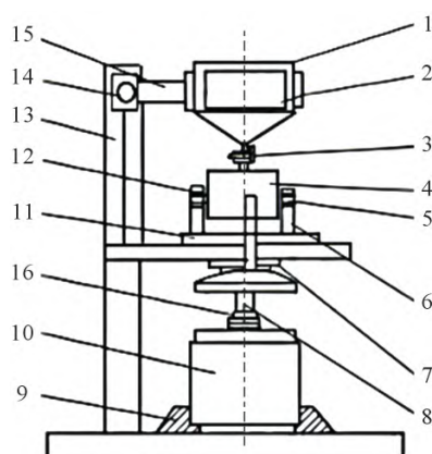
1- 熔化炉;2- 加热器;3- 开关阀;4- 铸型块;5- 铸型转轴 6- 铸型支架;7- 空间凸轮;8- 离心转轴;9- 电机架 10- 变速电机;11- 铸型转台;12- 轴承;13- 机座 14- 高度调节手轮;15- 支撑架;16- 联轴器
