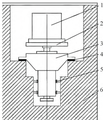
1- 离心模具;2- 工作盘;3- 机座;4- 纵向减振;5- 水平减振 6- 设备基础
