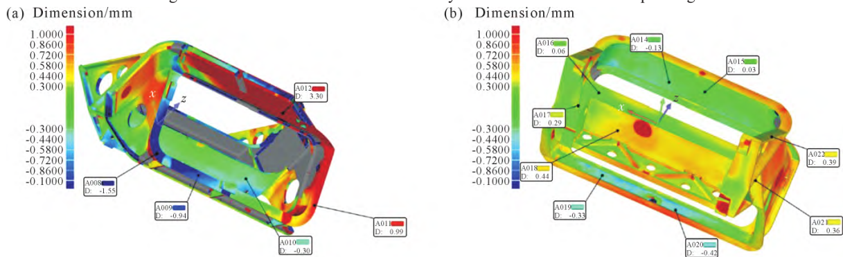
图 10 尺寸测量结果:(a) 顶注式;(b) 底注式
