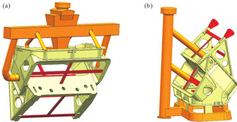
图2 浇注系统:(a)顶注式;(b)底注式
