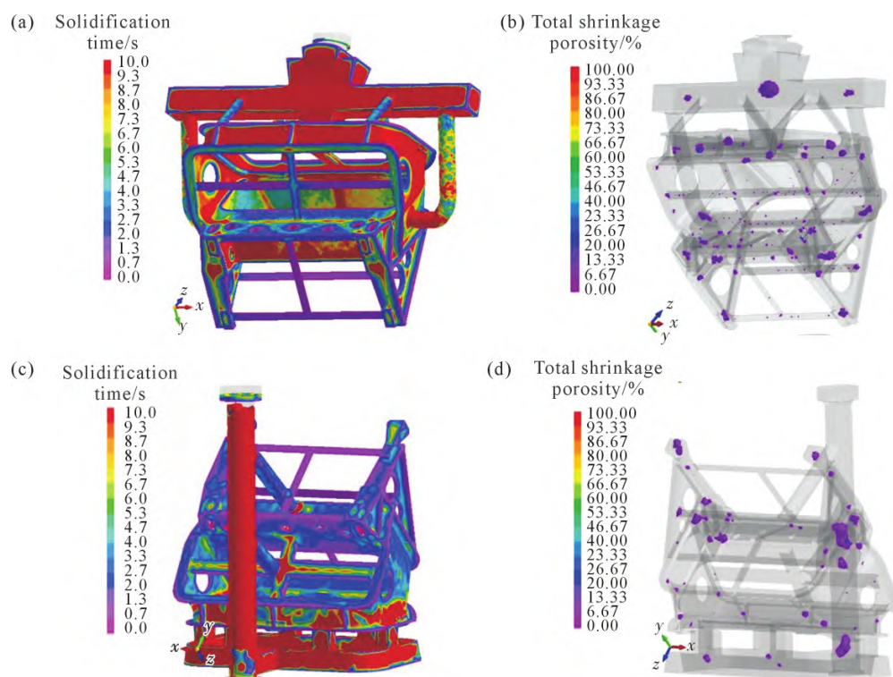
图 5 不同浇注方式下凝固时间及缺陷分布:(a, b) 顶注式;(c, d) 底注式
