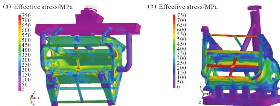
图 6 不同浇注方式下有效应力:(a) 顶注式;(b) 底注式
