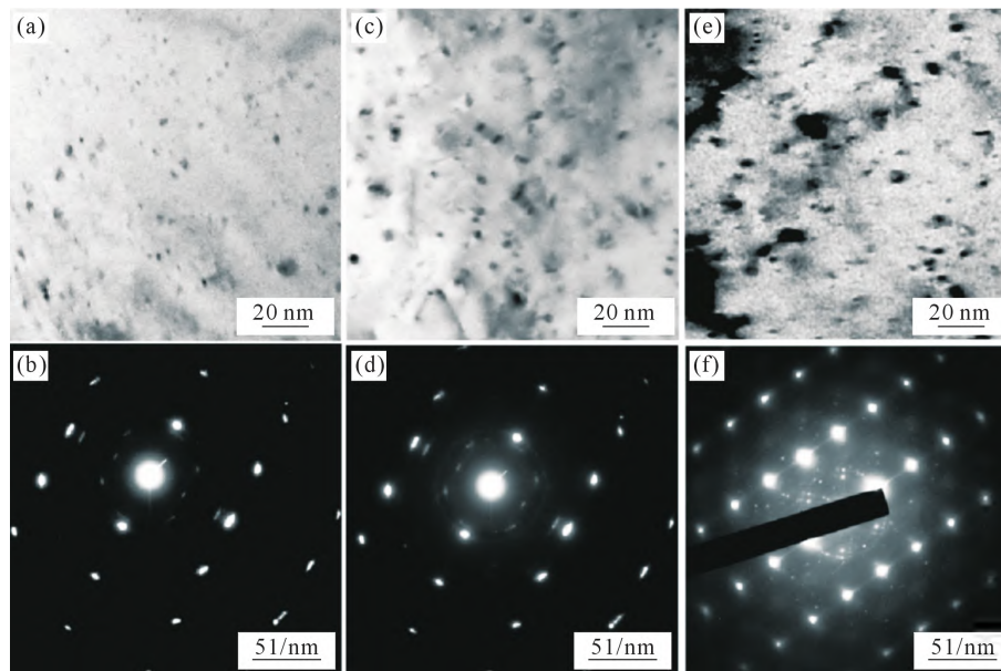
图 6 Cu-0.81Cr-0.12Zr-0.05La-0.05Y 合金在不同温度时效 60 min 时 TEM 图像和选区衍射图谱:(a~b) 450 °C, (c~d) 500 °C, (e~f) 550 °C [45]
