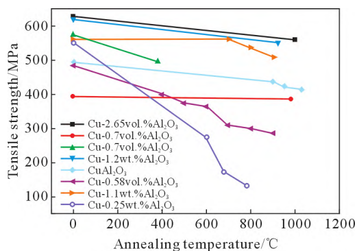
图 12 Cu-Al 2 O 3 合金强度随退火温度变化情况 [88,90,93-97]
