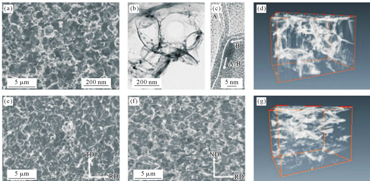
图 18 3D-GLNN/Cu 复合材料蚀刻 Cu 后 3D-GLNN 的 SEM 及 TEM 图像:(a~b) 热压 3D-GLNN/Cu 复合材料 3D-GLNN 的 SEM 及 TEM 图, (c) 3D-GLNN Y 型互连区域 HRTEM 图像, (d, g) 热压及热轧 3D-GLNN/Cu 复合材料 3D-GLNN 的 FIB-3D 重构结果, (e~f) 热轧 3D-GLNN/Cu 复合材料 3D-GLNN 沿 TD-RD 及 ND-RD 平面的 SEM 图像 [150]
