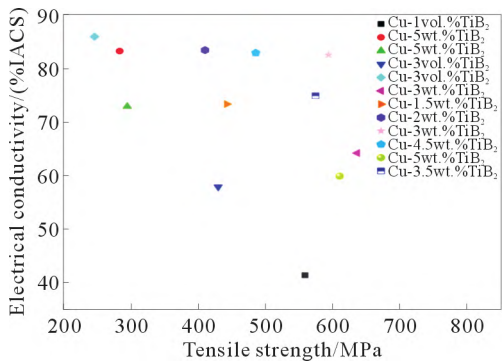
图 14 Cu-TiB 2 复合材料的抗拉强度和电导率比较 [100-102,105,107-113]
