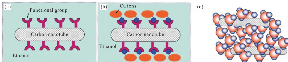
图 16 碳纳米管/铜复合粉末的分子级混合过程:(a) 在乙醇中制备官能化稳定的碳纳米管悬浮液,(b) 溶解铜盐,如 \text{Cu}(\text{CH}_3\text{COO})_2 , 并将 Cu 离子附着在碳纳米管表面的官能团上,(c) 通过加热使溶剂蒸发 [140]
