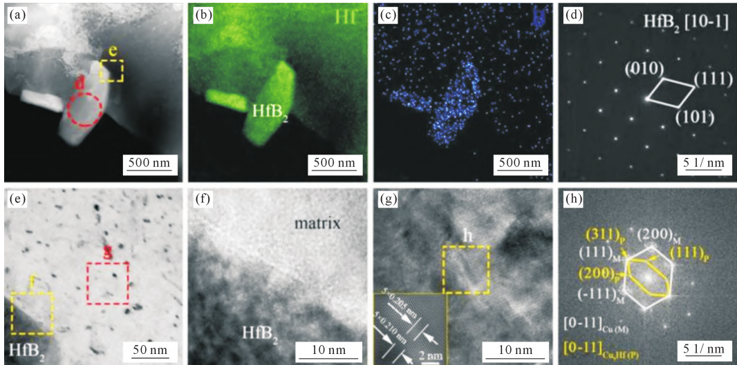
图 15 2HfB 2 /Cu-0.9Hf 复合材料的 STEM 表征:(a) HAADF 形貌,(b~c) 图(a)的 EDS 图,(d) 增强体的衍射斑点,(e) 图(a)放大图像的亮场像,(f) 图(e)增强体与基体界面处的 HRTEM,(g) 图(e)基体的 HRTEM,(h) 图(g)的 FFT [116]
