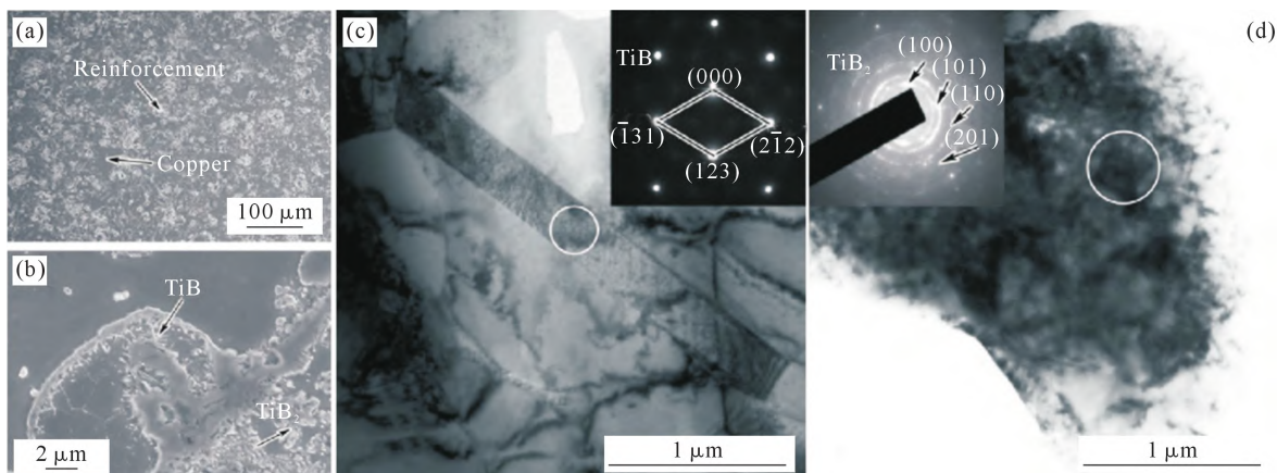
图 13 3%( \text{TiB}_2 +TiB)/Cu: (a~b) SEM 像, (c~d) TEM 亮场像及 SAED 图谱 [103]
