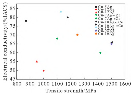
图 3 部分 Cu-Ag 合金的抗拉强度和导电性能 [9-10,14-18] Fig.3 Tensile properties and electrical conductivity of several Cu-Ag alloys [9-10,14-18]
