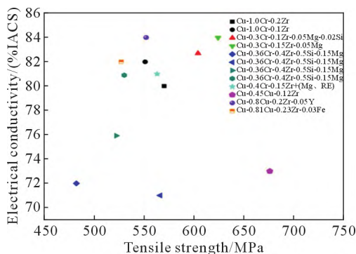
图 7 部分 Cu-Cr-Zr 合金的抗拉强度和导电性能 [52-59]
