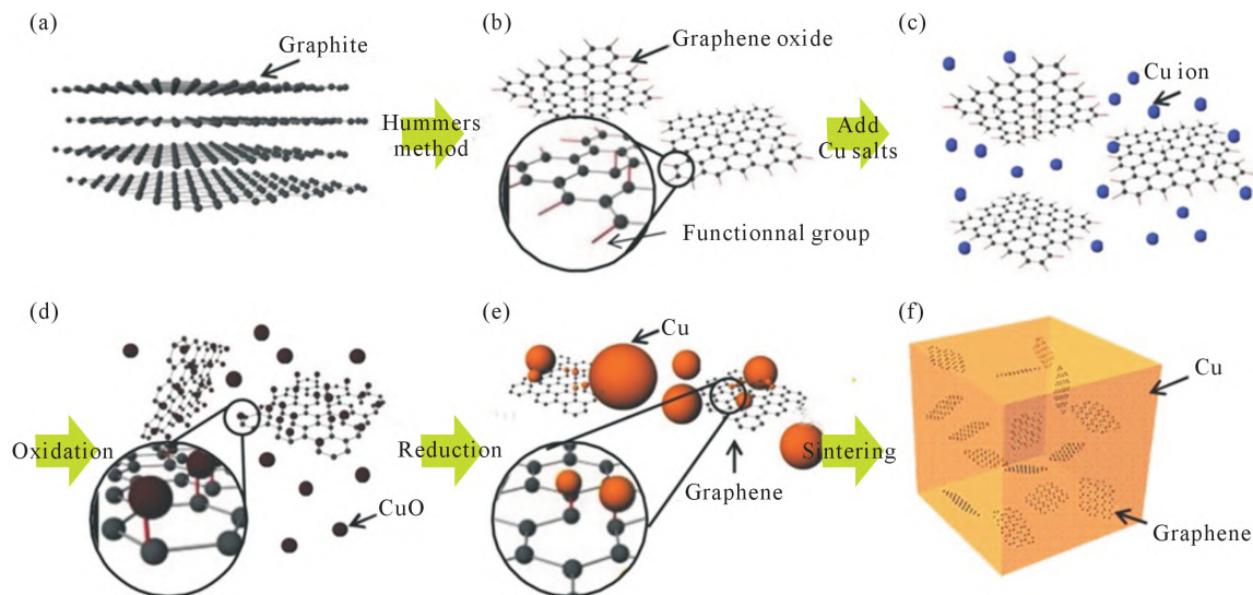
图 17 RGO/Cu 纳米复合材料的制备工艺示意图:(a) 原始石墨,(b) 用 Hummers 方法制备氧化石墨烯,(c) 铜盐在氧化石墨烯溶液中的分散,(d) 在氧化石墨烯上将 Cu 离子氧化为 Cu 氧化物,(e) 氧化铜和氧化石墨烯的还原,(f) 烧结还原氧化石墨烯/Cu 纳米复合粉体 [146]
