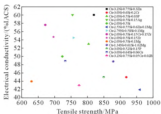
图 4 部分 Cu-Ni-Si 合金的抗拉强度和导电性能 [26,31-40]
