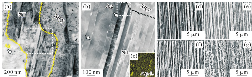
图 2 不同热处理条件下合金的 SEM 图:(a~c) 时效处理后 DPD Cu-5%Ag 样品的 TEM 明场像, STEM-HAADF 图像及纳米孪晶区域的 Ag 元素分布,(d~g) Cu-12Ag 纵断面 SEM 图及在不同退火条件(200 °C/185 h, 300 °C/209 h, 400 °C/190 h)下的 SEM 图 [9-10]
