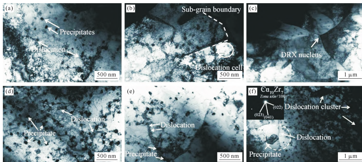
图 5 不同 Zr 含量的 Cu-Ni-Si-Co-Zr 合金在 0.002 s -1 、800 °C 变形时的微观形貌:(a~c) 0.036%Zr, (d~f) 0.084%Zr [43]
