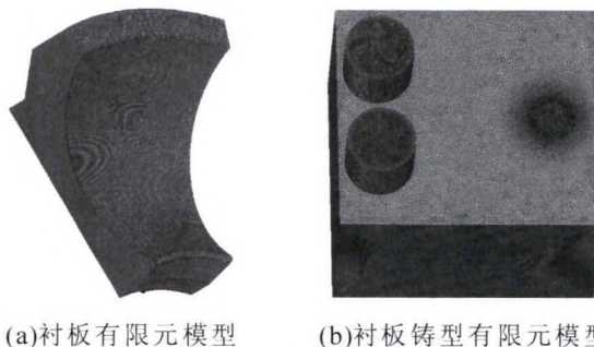
(a)衬板有限元模型 (b)衬板铸型有限元模型 图 3 衬板及其铸型有限元模型 Fig.3 Typical lining casting and casting finite element model
