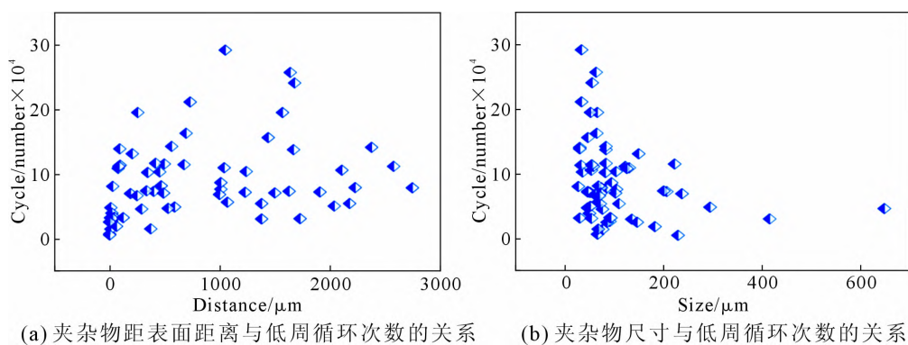
图2 夹杂物距表面距离和尺寸与低周循环次数的关系
