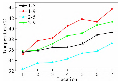
图 11 不同位置水路温度分布
