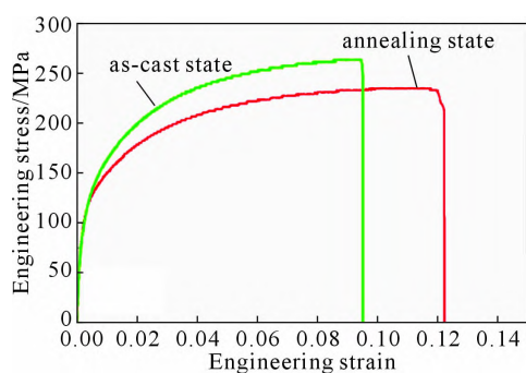
图5 AlSi7MgMn 压铸态和退火态工程应力-应变曲线
