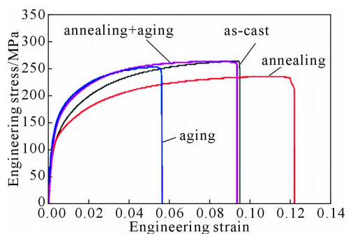
图10 不同工艺条件下高压铸造 AlSi7MgMn 铝合金的工程应力-应变曲线
