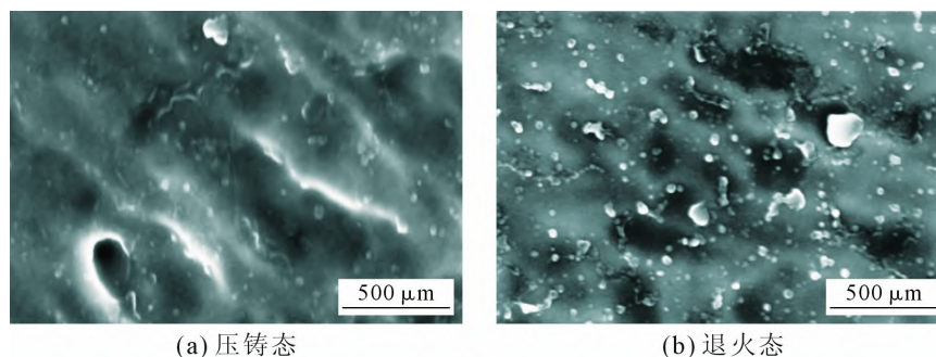
图4 压铸态和退火态 AlSi7MgMn 合金 \alpha -Al 基体上纳米尺寸 Si 颗粒形貌图
