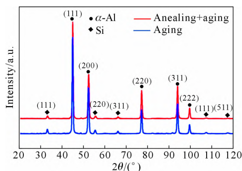
图6 时效态和退火时效态 AlSi7MgMn 合金 X 射线衍射图谱
