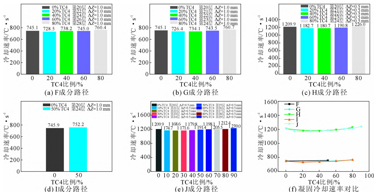
图5 不同成分路径的凝固冷却速率及其对比
