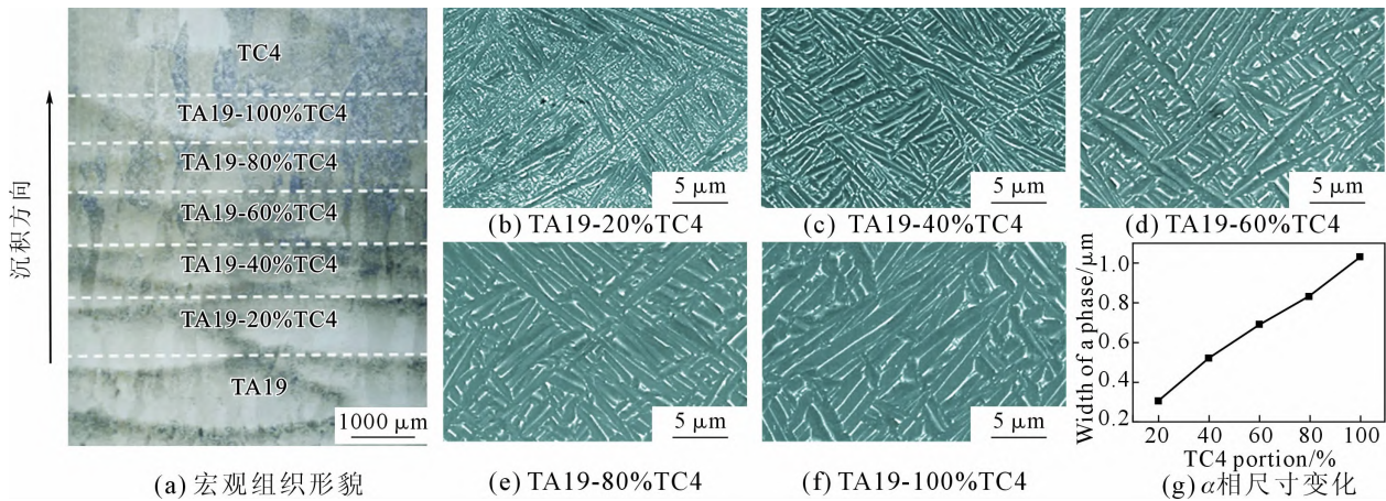
图 7 G 成分路径梯度试样过渡区宏观、微观和电镜组织形貌图
