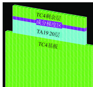
图 1 TC4-TA19 功能梯度材料模型示意图
