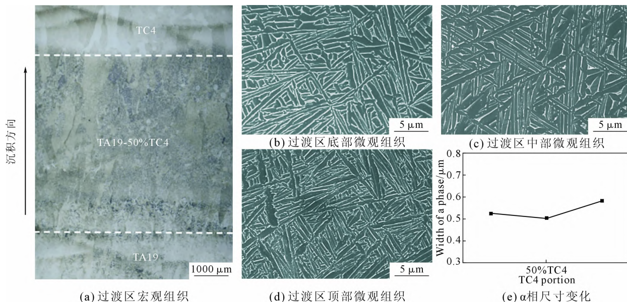
图6 I成分路径梯度试样过渡区宏观、微观和电镜组织形貌图
