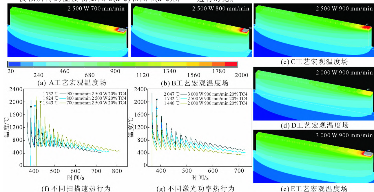
图 2 不同激光功率和扫描速度下成分梯度区第 1 层的宏观温度场示意图和熔池热行为曲线
