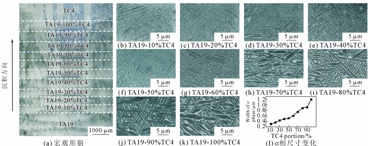
图 8 J 成分路径梯度试样过渡区宏观微观和电镜组织形貌图
