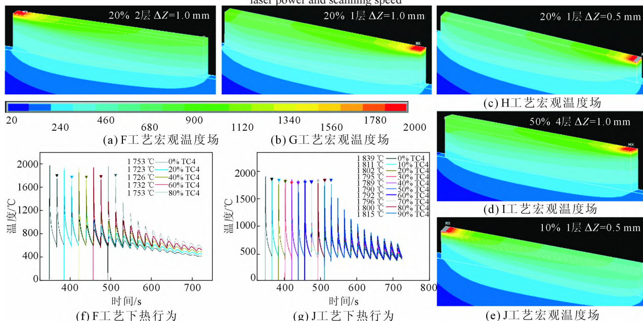
图 3 不同成分路径下成分梯度区第 1 层的宏观温度场和部分熔池的热行为曲线
