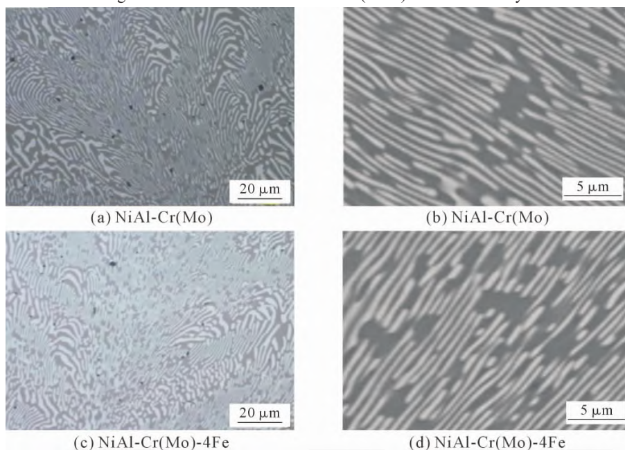
图 4 1\ 200\ ^\circ\text{C}/36\ \text{h} (HT-3)热处理合金的显微组织
