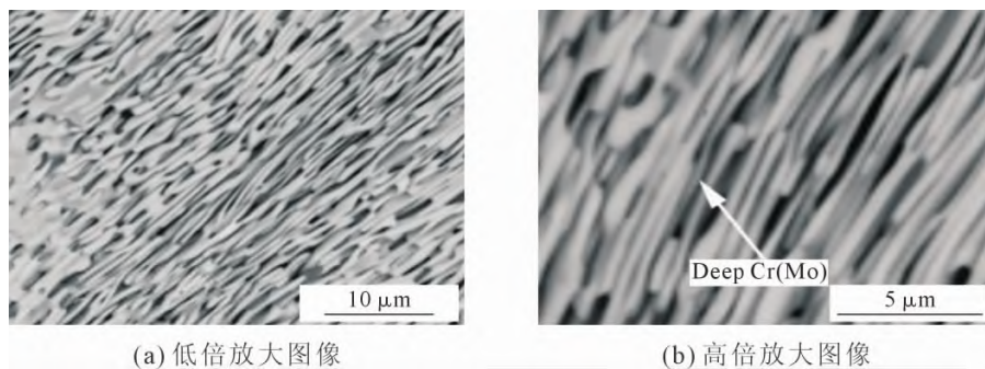
图 5 深度腐蚀 NiAl-Cr(Mo)-4Fe 共晶合金在 1\ 200\ ^\circ\text{C}/36\ \text{h} (HT-3)下的显微组织 Fig.5 Microstructure of deeply corroded NiAl-Cr(Mo)-4Fe eutectic alloys at 1\ 200\ ^\circ\text{C}/36\ \text{h} (HT-3)
