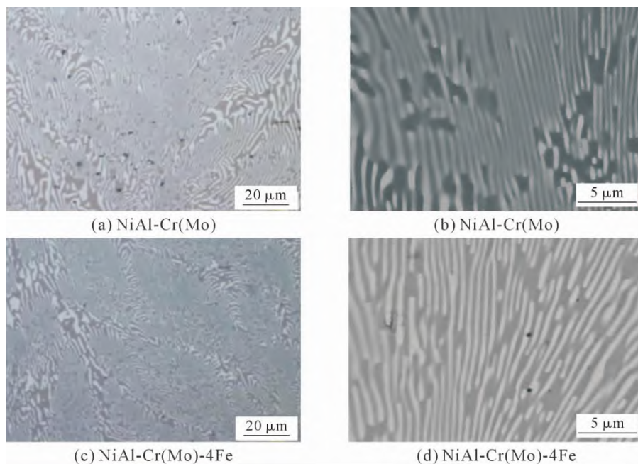
图 3 1\ 200\ ^\circ\text{C}/12\ \text{h} (HT-2)热处理合金的显微组织
