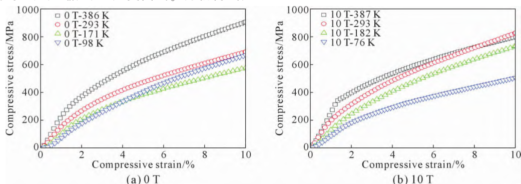
图 3 有无磁场下 CrCoNi 合金以不同过冷度凝固后的室温压缩应力-应变曲线
