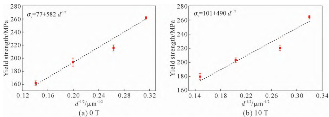
图4 有无磁场不同过冷度下 CrCoNi 合金抗压屈服强度与晶粒尺寸的关系
