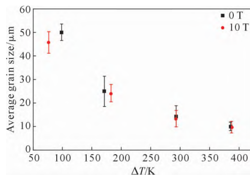
图 2 有无磁场下 CrCoNi 合金不同过冷度凝固的晶粒尺寸
