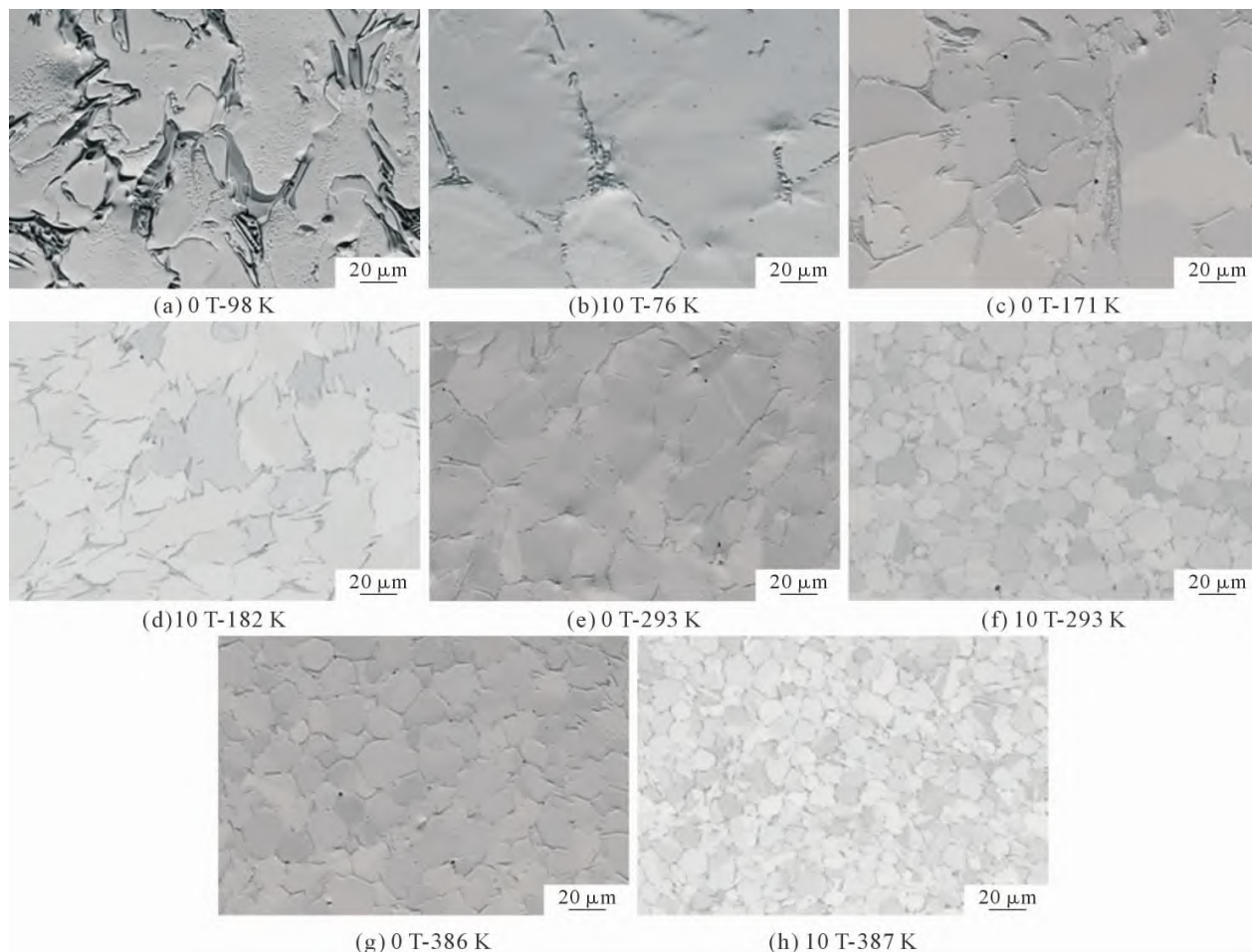
图 1 有无磁场不同过冷度下 CrCoNi 合金的微观组织
